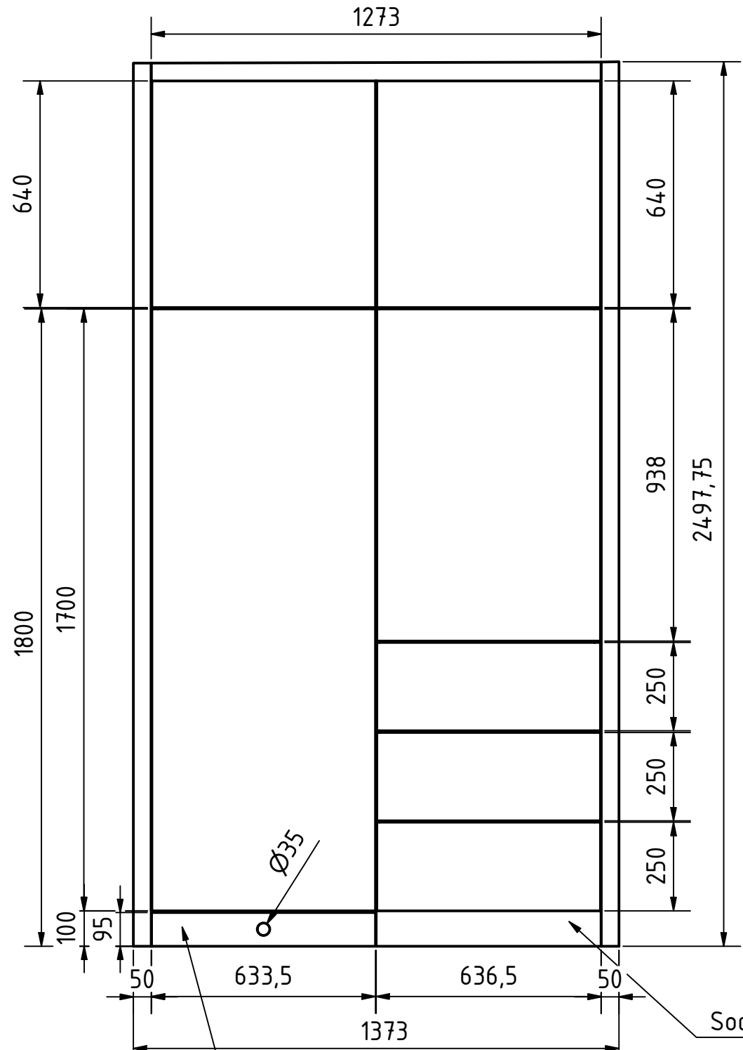
Ansicht mit Passleisten
